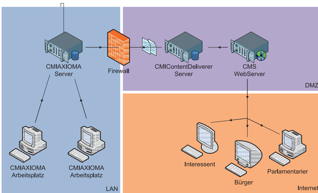
Systemarchitektur CMIAXIOMA-Publikator
