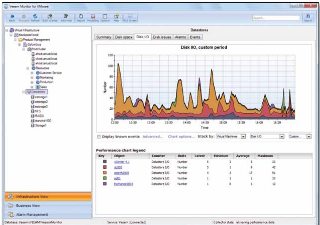
Veeam Monitor für eine konzentrierte Sicht auf die Monitoring-, Alarm- und Berichtsdaten der VMs
